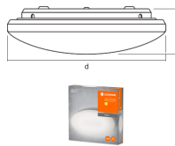
Technische Daten Ledvance LED-Wand- und Deckenleuchte Orbis Pure 400 h 24W 830 1800lm Weiß IP20
